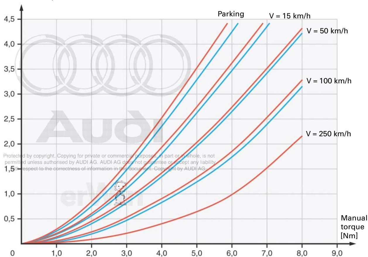
V187-Motor torque [Nm]
