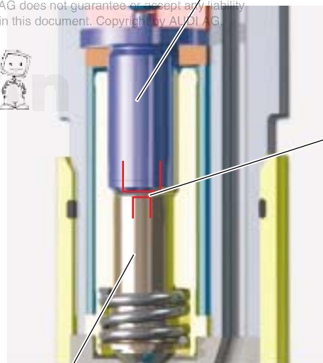
Coupler module
