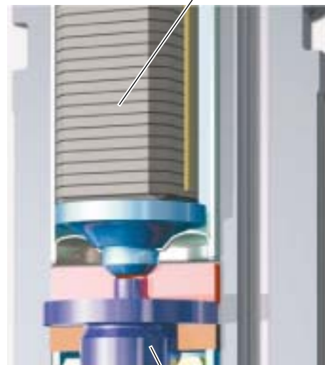
Actuator module
