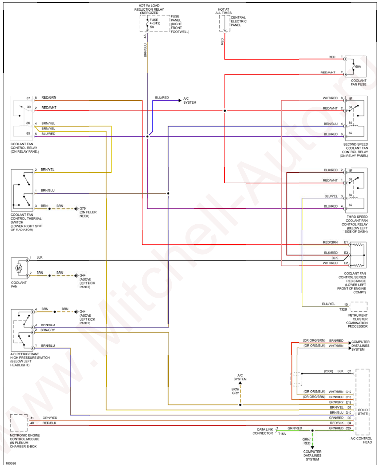
Fig. 7: Cooling Fan Circuit
